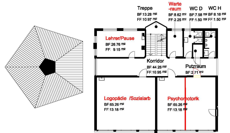
1. Obergeschoss
